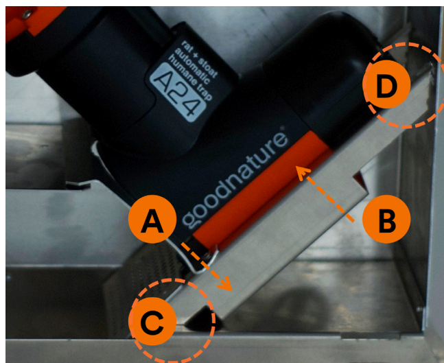
Bild 2: Montering på ingångsplattan.
